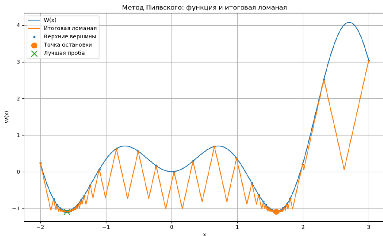
Рис 2 – График исходной функции и итоговой ломаной метода Пиявского
