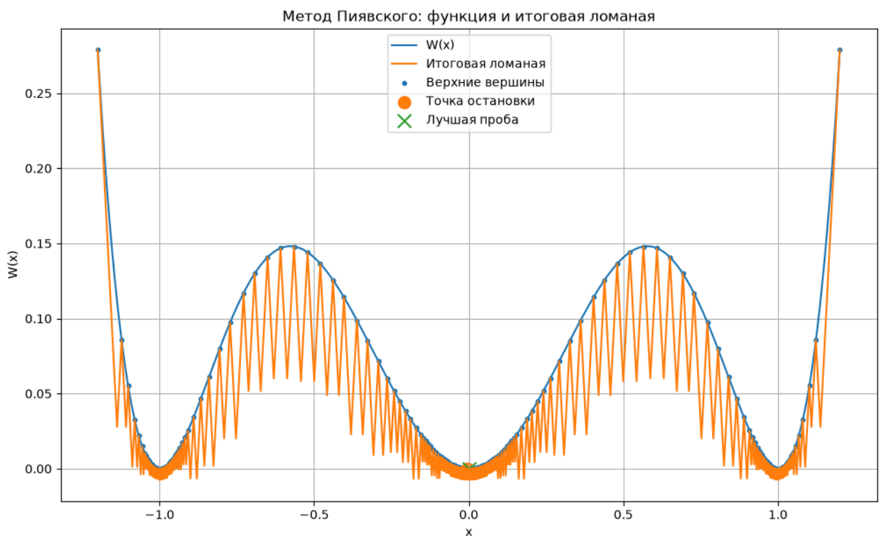
Рис 4 – График дополнительной функции и итоговой ломаной метода Пиявского
